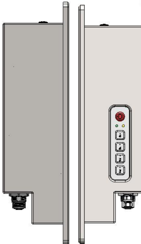
Side View (MPPC1001PC)
